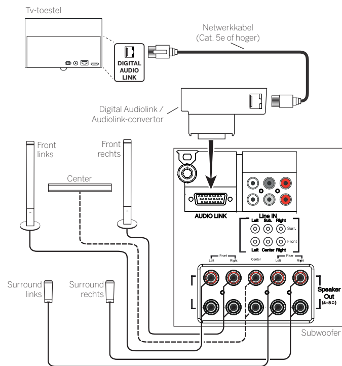
Voorbeeld voor de aansluiting van een luidsprekersysteem (Subwoofer met AUDIO LINK) aan het tv-toestel
