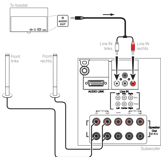
Voorbeeld voor de aansluiting van een luidsprekersysteem aan het tv-toestel
