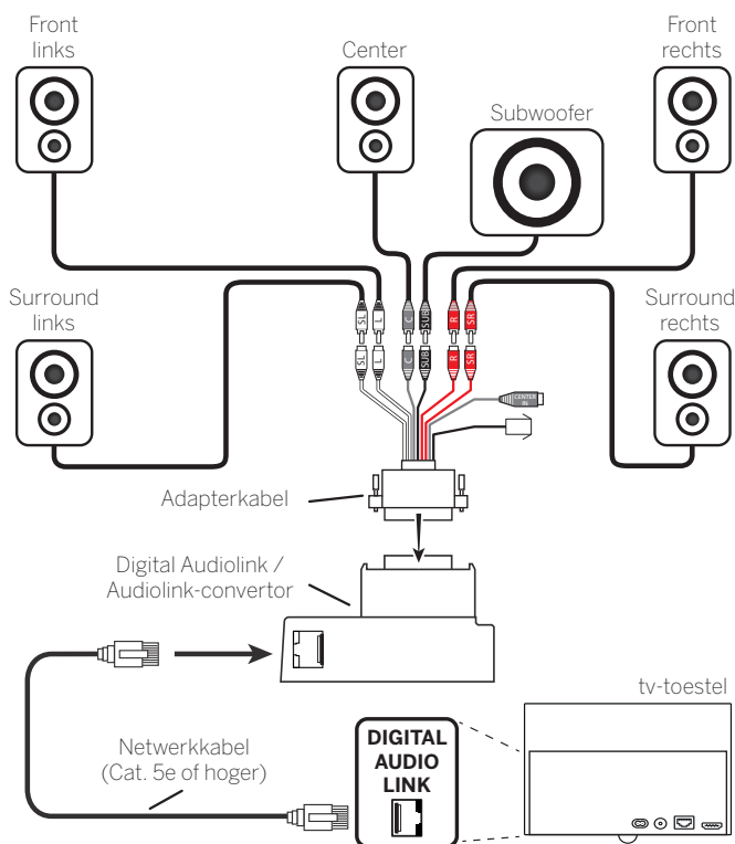
Aansluiting van actieve luidsprekers op het tv-toestel
