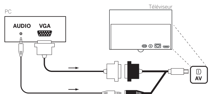
Exemple de raccordement d'un PC
