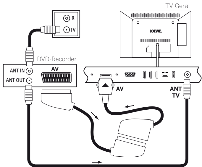
Anschlussbeispiel eines DVD-Recorders
