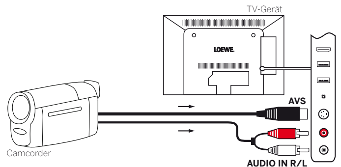
Anschlussbeispiel eines Camcorders
