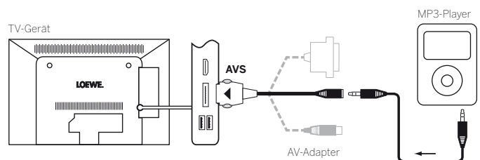
Anschlussbeispiel eines MP3-Players
