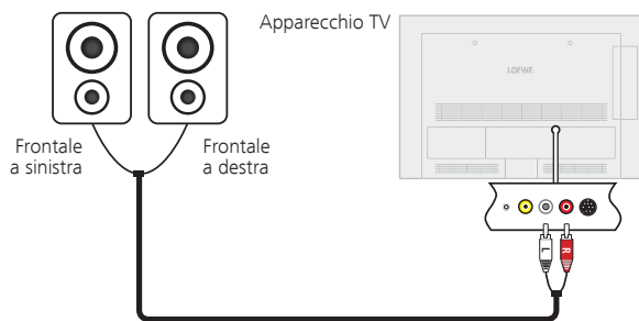
Connessione degli altoparlanti attivi all'apparecchio TV
