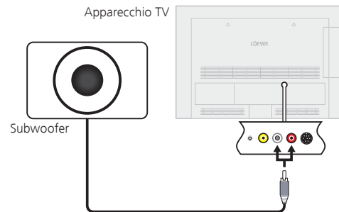
Collegamento di un subwoofer all'apparecchio TV
