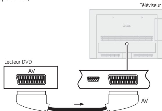
Exemple de raccordement d'un lecteur de DVD
