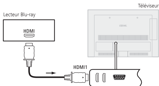
Exemple de raccordement d'un appareil HDMI (par ex., lecteur Blu-ray)
