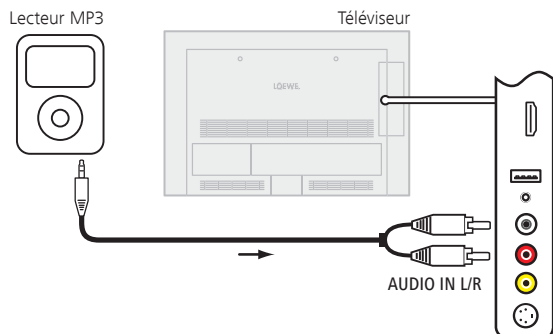
Exemple de raccordement d'un lecteur MP3
