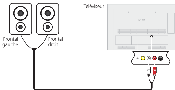
Raccordement de haut-parleurs actives au téléviseur
