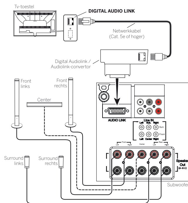
Voorbeeld voor de aansluiting van een luidsprekersysteem aan het tv-toestel
