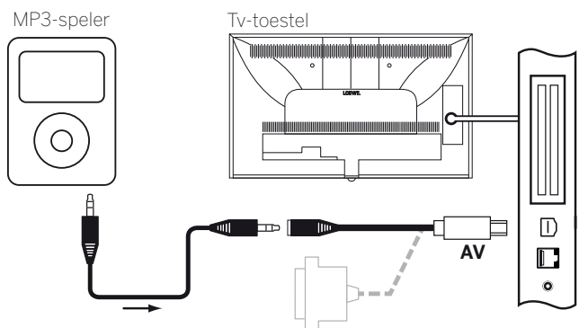
Aansluitvoorbeeld van een MP3-speler
