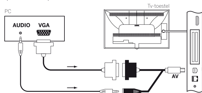
Aansluitvoorbeeld van een pc
