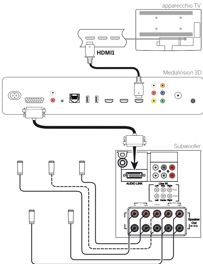
Collegamento del sistema audio al televisore
