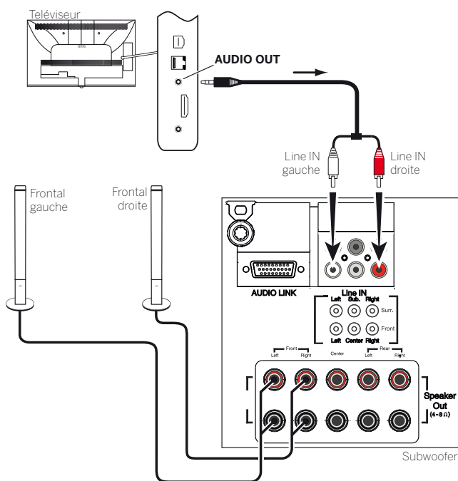
Exemple de raccordement d'un système de haut-parleurs sur le téléviseur
