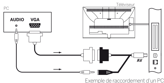
Exemple de raccordement d'un PC
