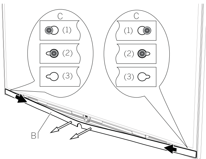
C (1) Placa frontal (B) del televisor, cierre en bayoneta (C) bloqueado C (2) Placa frontal (B) del televisor, cierre en bayoneta (C) desbloqueado C (3) Placa frontal (B) retirada
