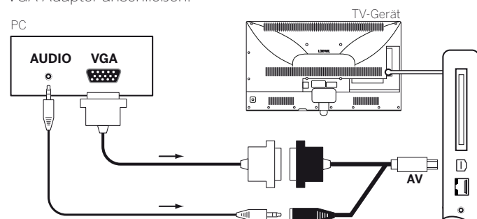
Anschlussbeispiel eines PC
