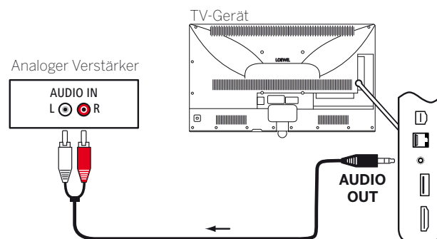
Beispiel für den Anschluss eines Lautsprechersystems an das TV-Gerät
