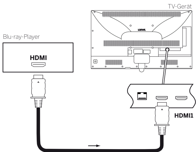
Anschlussbeispiel eines HDMI-Gerätes (z.B. Blu-ray-Player)
